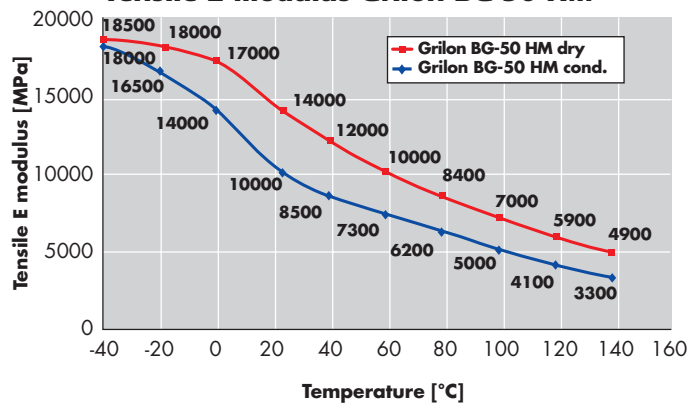
Tensile E modulus Grilon BG-50 HM
