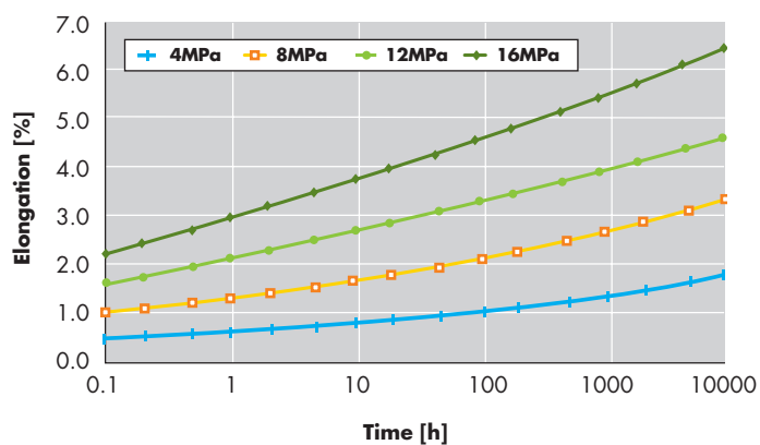
Creep curves Grilon TSS at 23°C / 50% r.h.
