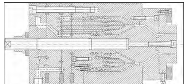
Fig. 2: Spiral mandrel die system from ETA Kunststofftechnologie GmbH
